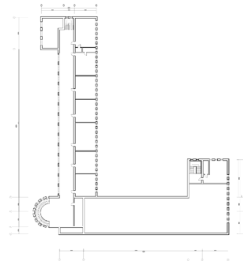
TREČIO AUKŠTO PLANAS
