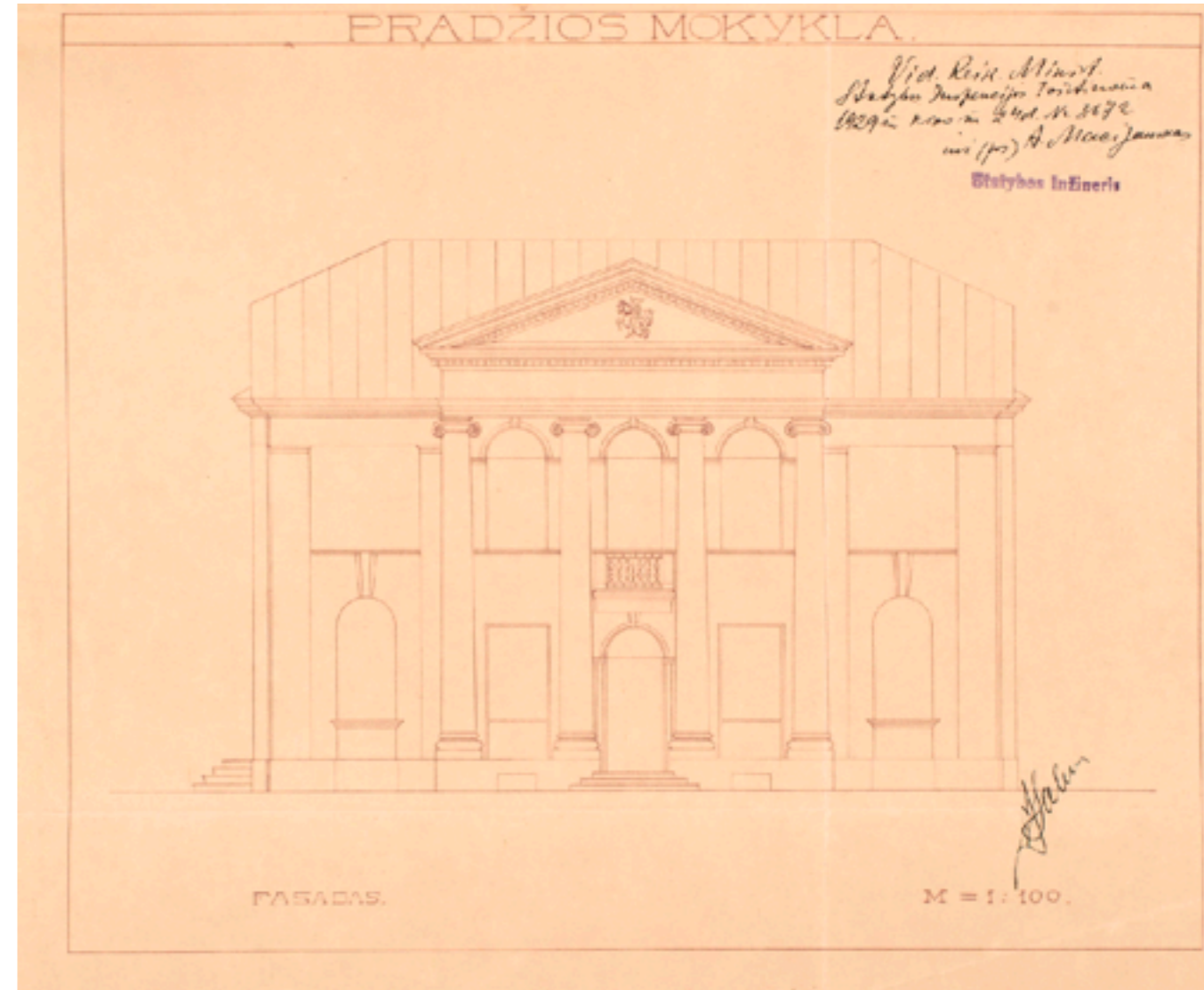
pagrindinis fasadas
