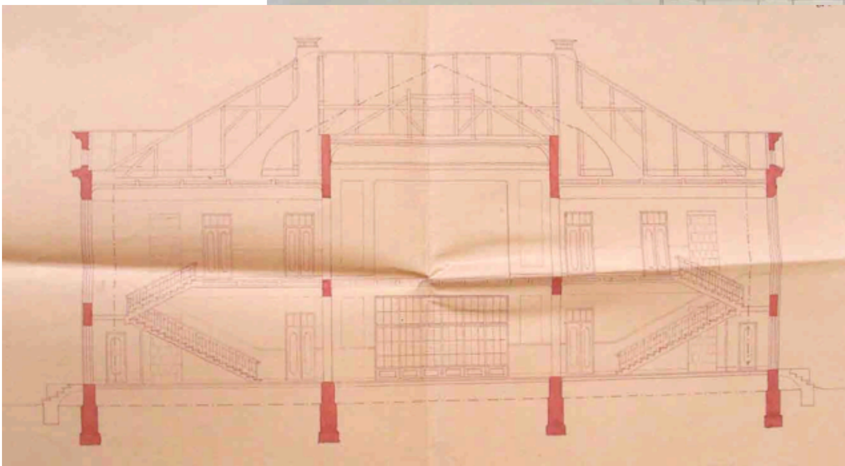
Švēkšnos "Saulis" gimnazijas pagrindinis fasadas ir pjūvis, 1925 m.
