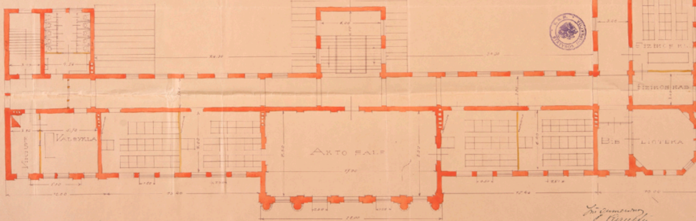
antrojo aukšto planas
