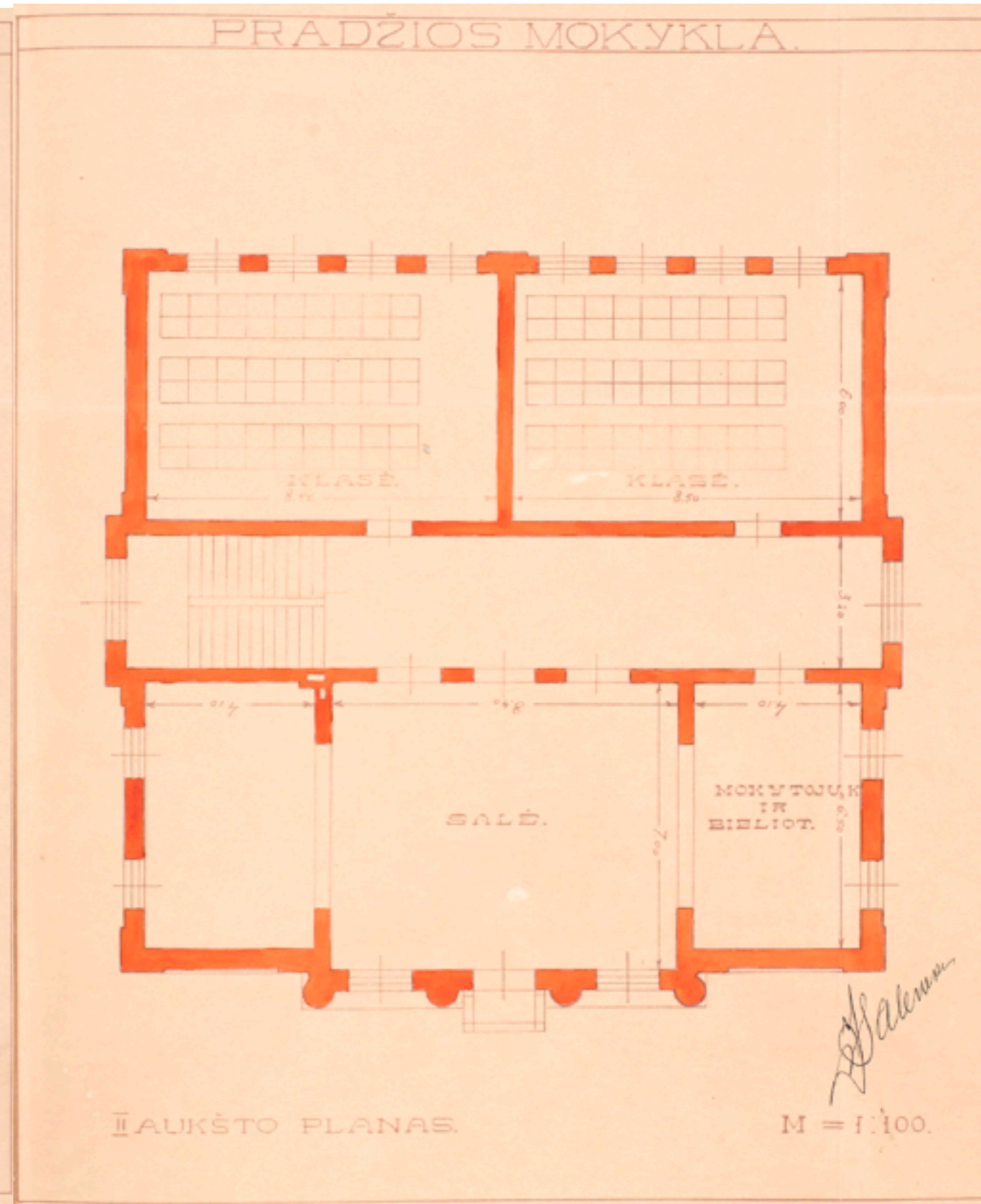
antrojo aukšto planas
