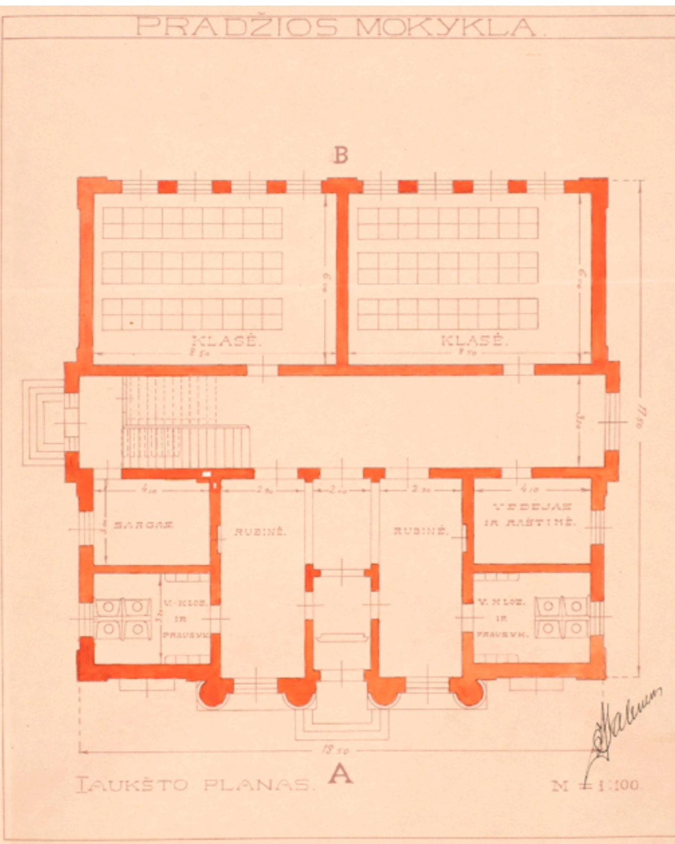
pirmojo aukšto planas
